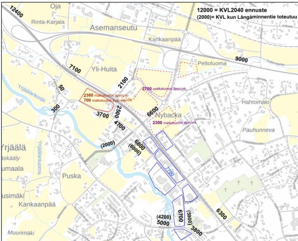
Kuva 5.1: Tarkistettu liikenne-ennuste
