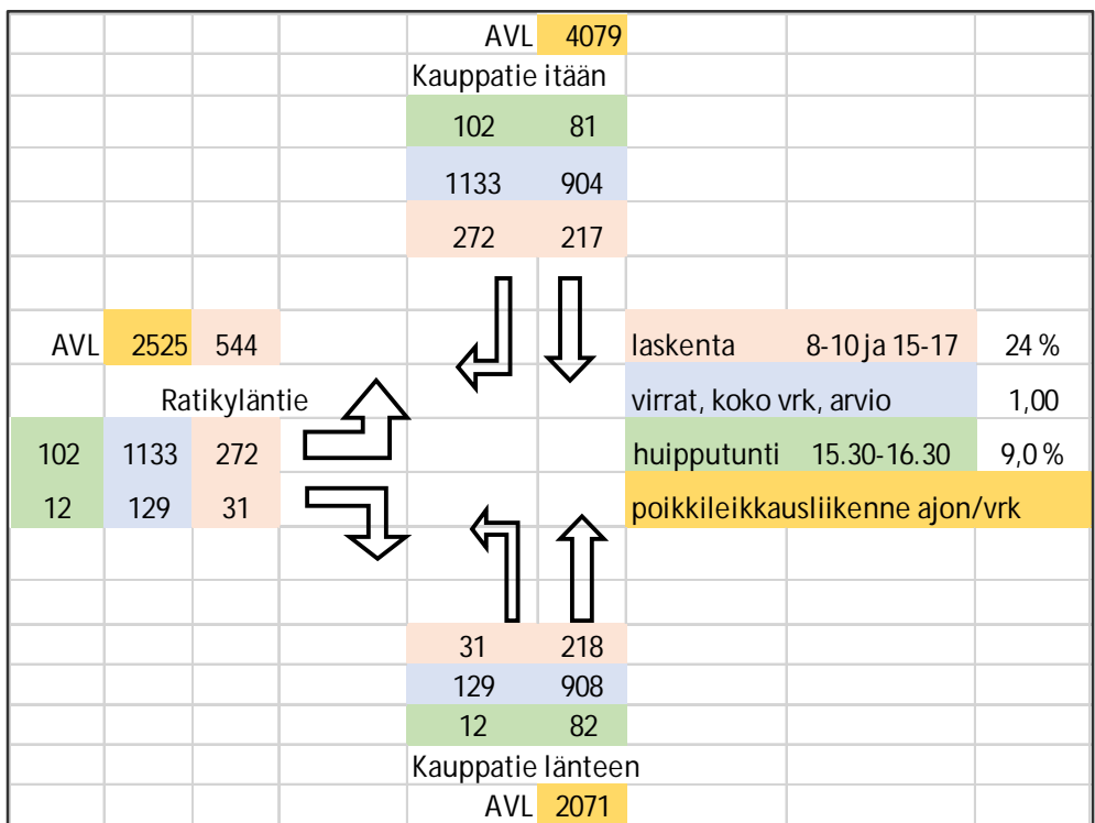
Kuva 4.4: Ratikylän/Kauppätien risteys, liikennelaskennan 2020/8 tulos.
