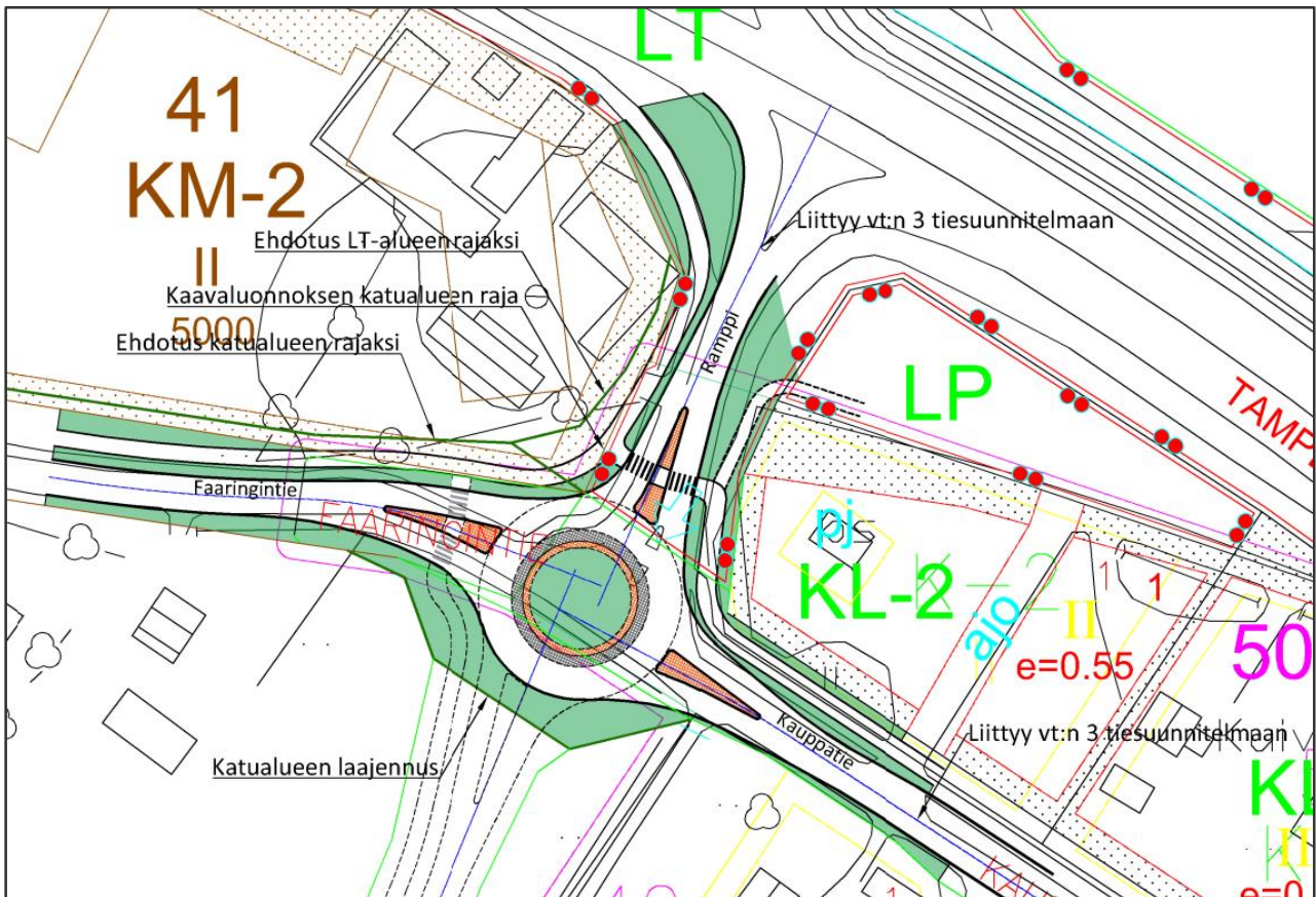
Kuva 12: Luonnos kiertoliittymäksi ja sen tilantarve Rampin, Faaringintien ja Kauppaticien liittymässä.
