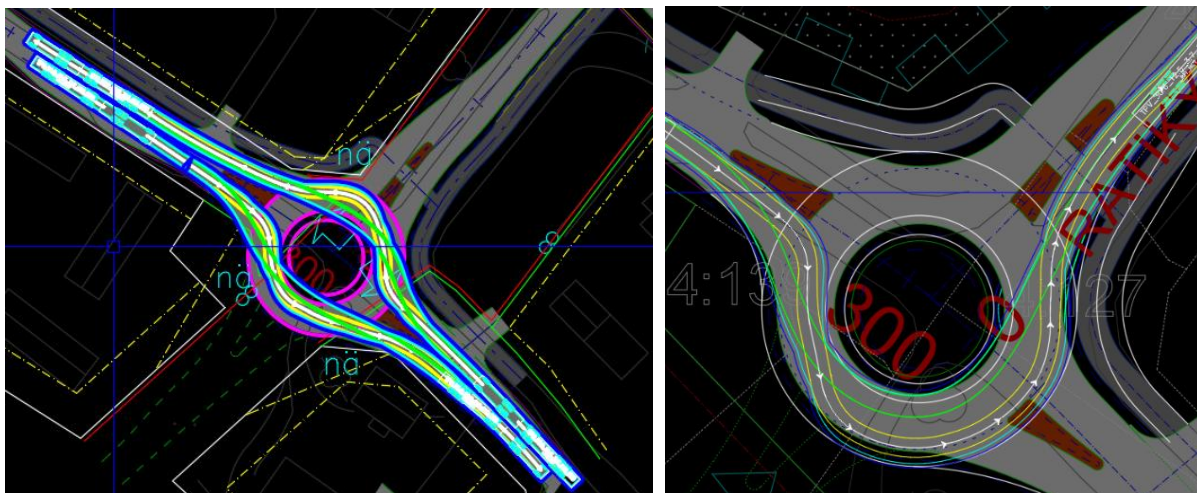
Kuva 11: HCT-ajourat ovat Kauppap tien suunnassa tiukat ja vaikeasti ajettavat, mutta juuri ja juuri mahdolliset (vasen kuva), ajo Ratikyläntieltä Kauppap tielle tai muut kääntyvät suunnat edellyttävät toimenpiteitä (oikealla oleva kuva).
