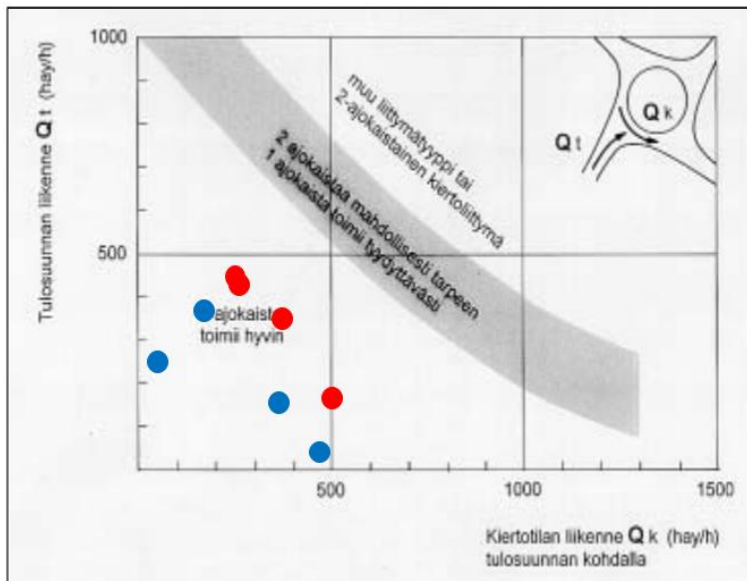
Kuva 10: Ratikyläntien/Kauppap tien kiertoliittymän välityskyky tasoliittymät-ohjeen mukaan, sinisellä Faaringintien/rampin liittymä ja punaisella Ratikyläntien liittymän tiedot.
